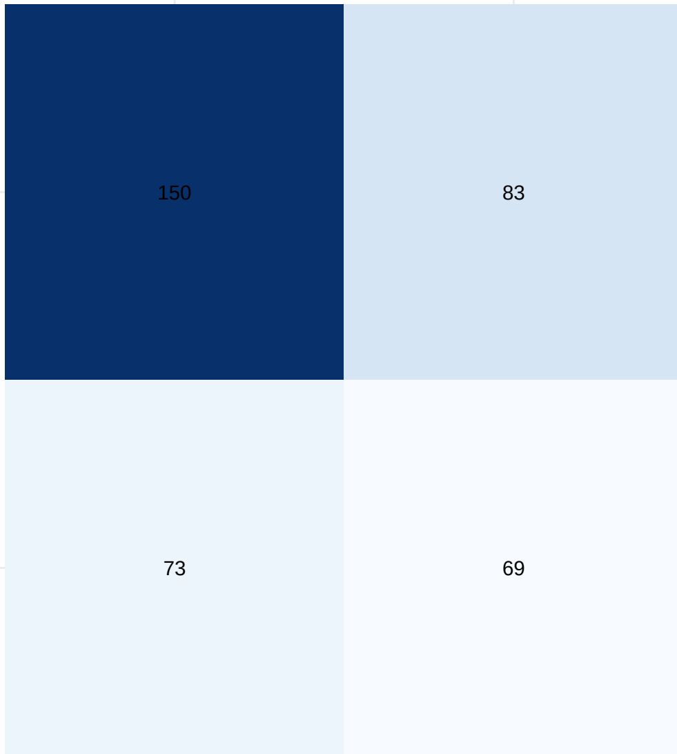
Matriz de confusión – KNN (k = 7)
