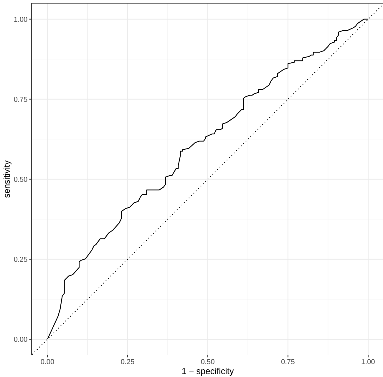
Curva ROC – KNN (k = 7)
