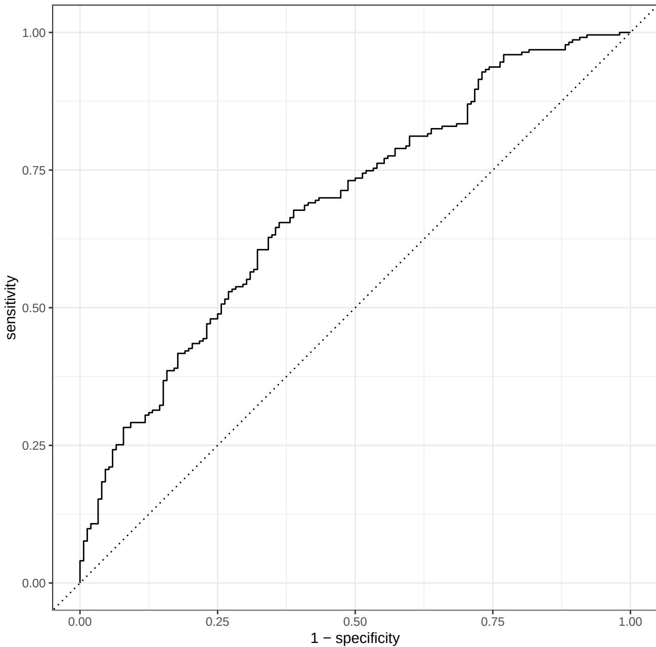
Curva ROC – KNN tuneado (k = 151)
