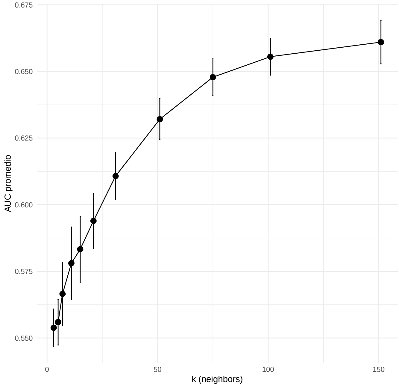
AUC promedio por valor de k (validación cruzada 5-fold)
