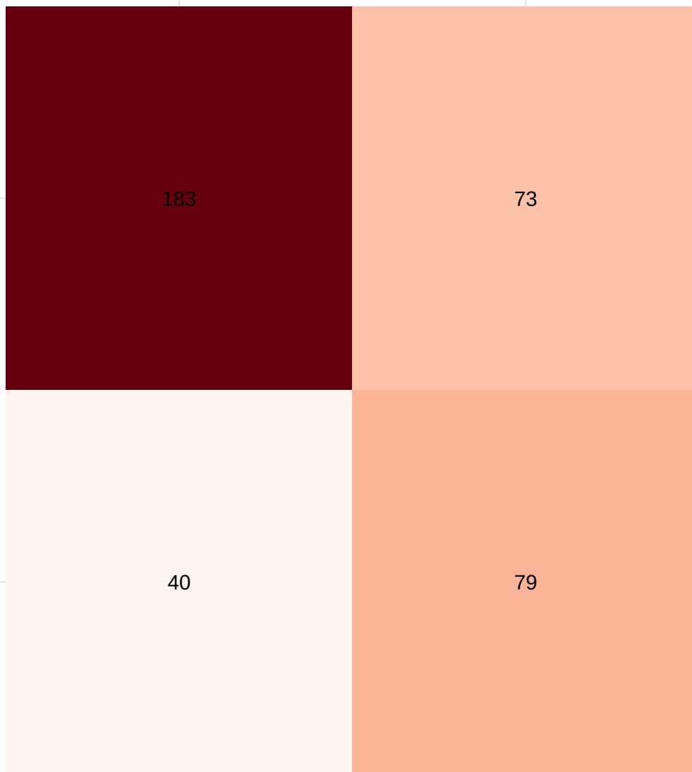
Matriz de confusión – Workflow Regresión Logística
