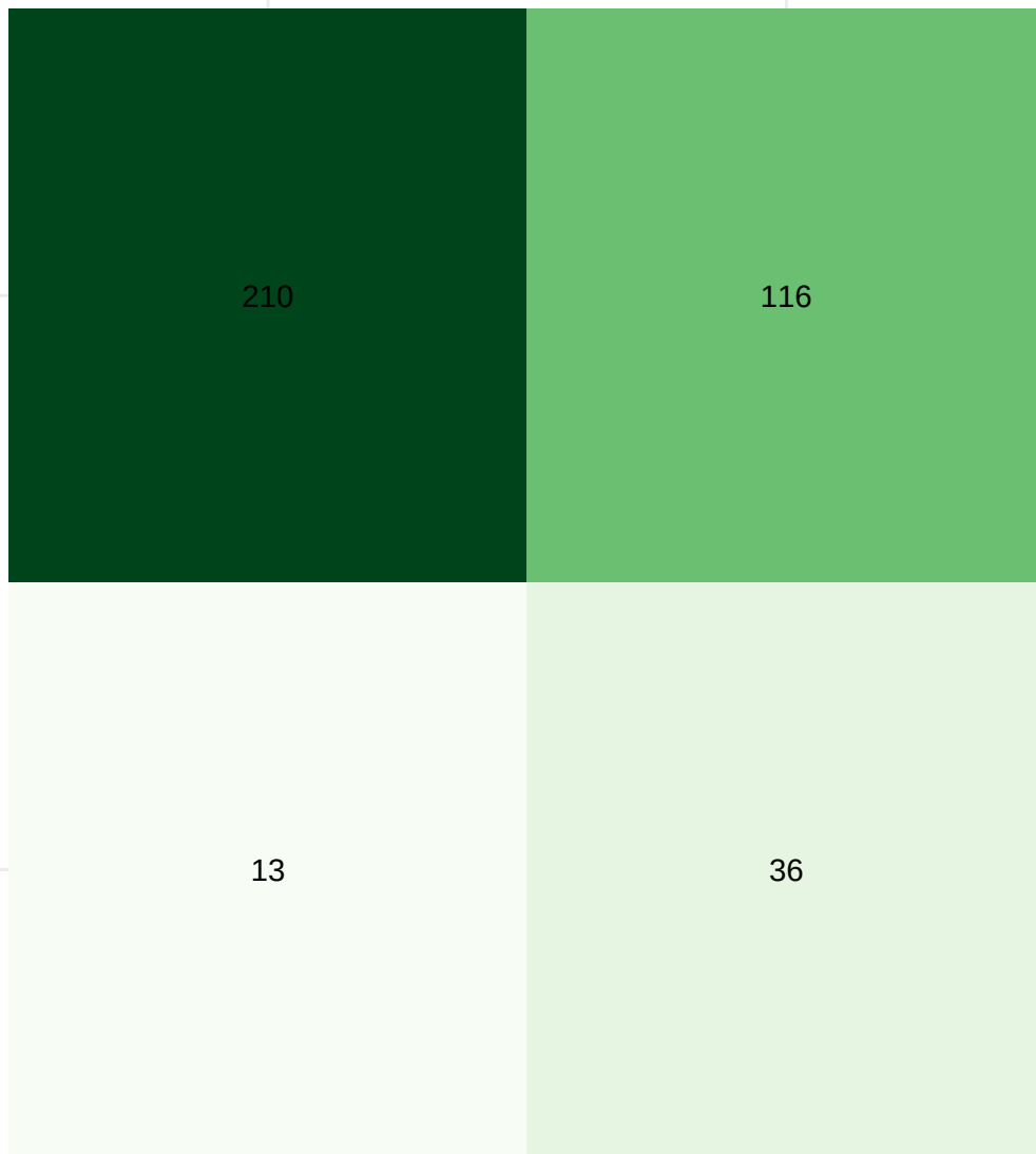
Matríz de confusión – KNN tuneado (k = 151)
